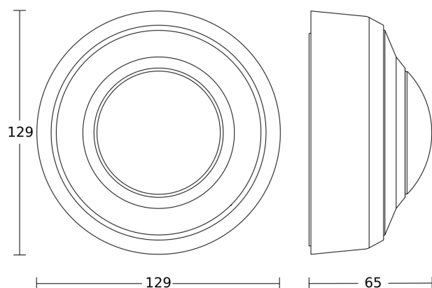
Dibujo acotado
